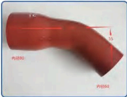
连接硅胶管
